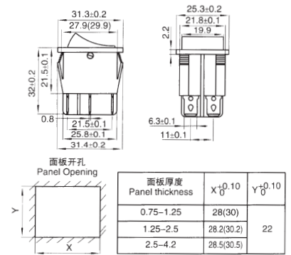
KCD4-202/4P
