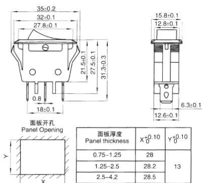
KCD3-201PV
