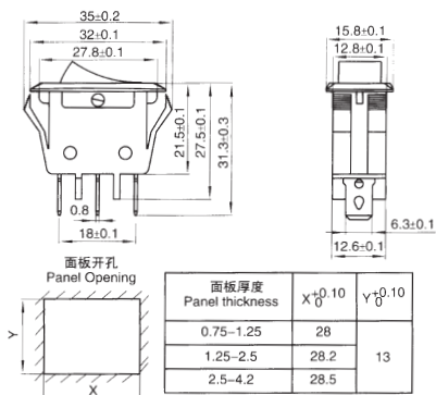
KCD3-201NC
