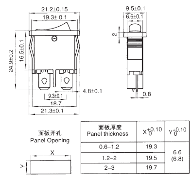
KCD1-110/2P
