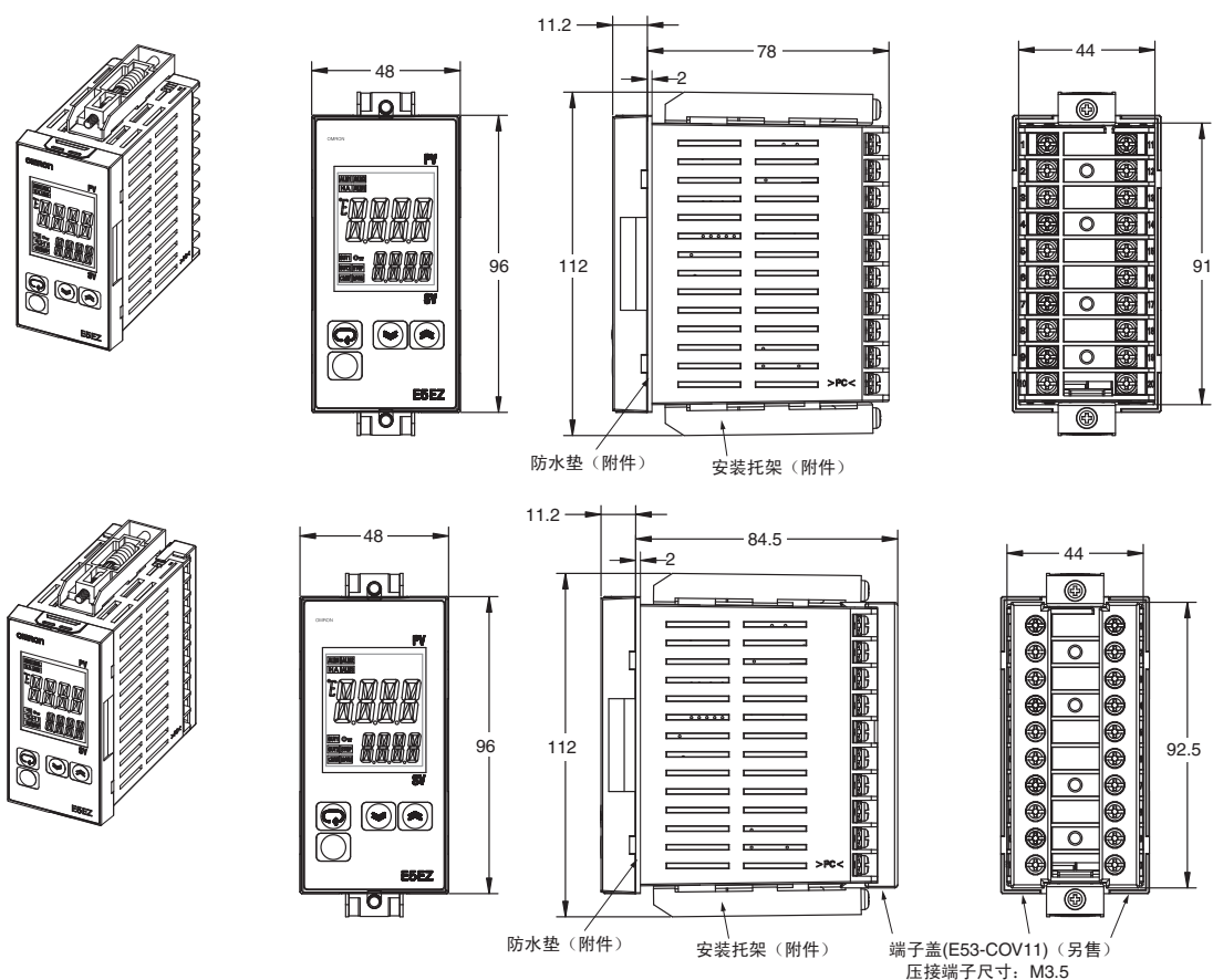
仪器面板尺寸
