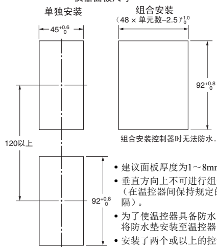
仪器面板尺寸
